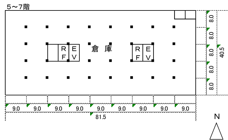
■ 平立図面
